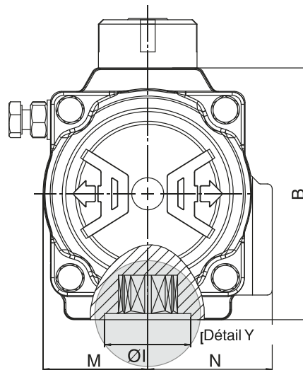
Type 0015U-1200U
