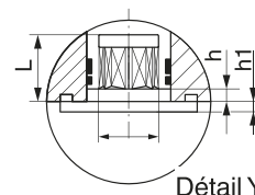
Type 5000U
