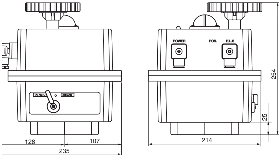
Type d'actionneur - J2140 et J2300
