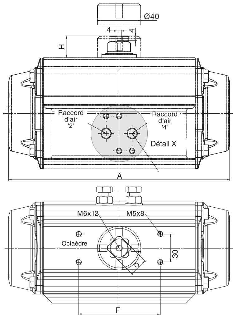
Type 0015U-1200U
