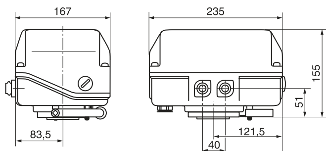
Type d'actionneur 2070
