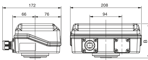
Type d'actionneur 3035
