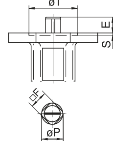
Forme de l'axe avec clavette DN 700 - 1200
