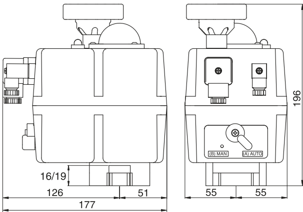
Type d'actionneur - J2140 et J2300
