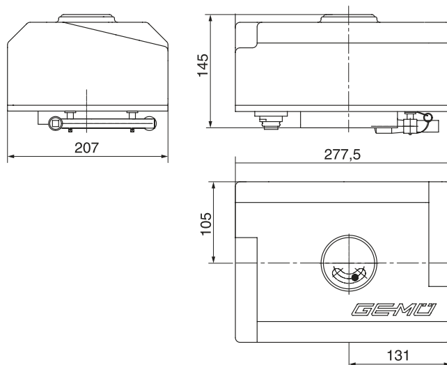
Type d'actionneur 4100, 4200
