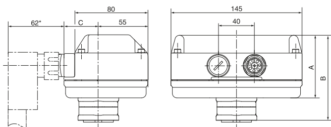
Type d'actionneur 1015, 2015
