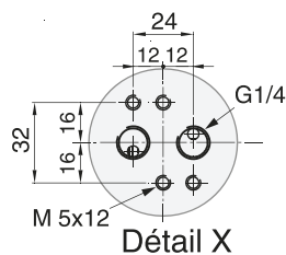
ADA/ASR 0020U-1750U
