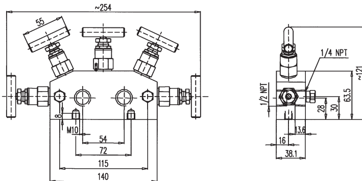
Manifold 5 voies
