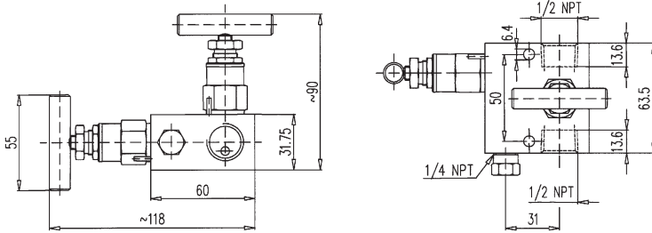
Manifold 2 voies
